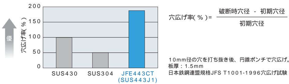
穴広げ特性
